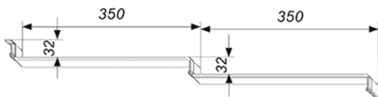
Rzut z boku
